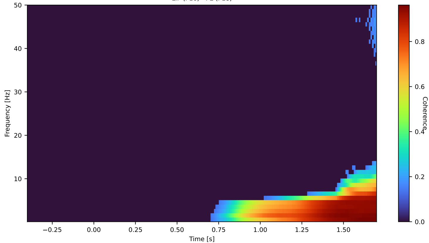
LIP (P16) - PE (P18)
